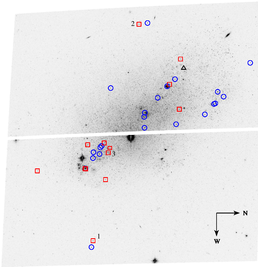
Рис. 1. Изображение галактики NGC 4068 в фильтре F606W на ACS/WFC-снимке космического телескопа им. Хаббла. Размер снимка 3.5 \times 3.5 . Север справа, восток вверх. Обозначения следующие: красные квадраты — красные сверхгиганты высокой металличности, синие кружки — голубые сверхгиганты, яркость которых превышает яркость сверхгиганта с эмиссионными линиями; черный треугольник — голубая звезда с эмиссионными линиями, которую изучали Yarovova et al. (2023). Можно отметить, что высокометаллические звезды не концентрируются в одной области, а распределены по всему телу галактики. Цифры 1, 2 и 3 маркируют звезды, которые обсуждаются далее (см. рис. 10 и раздел 4).
